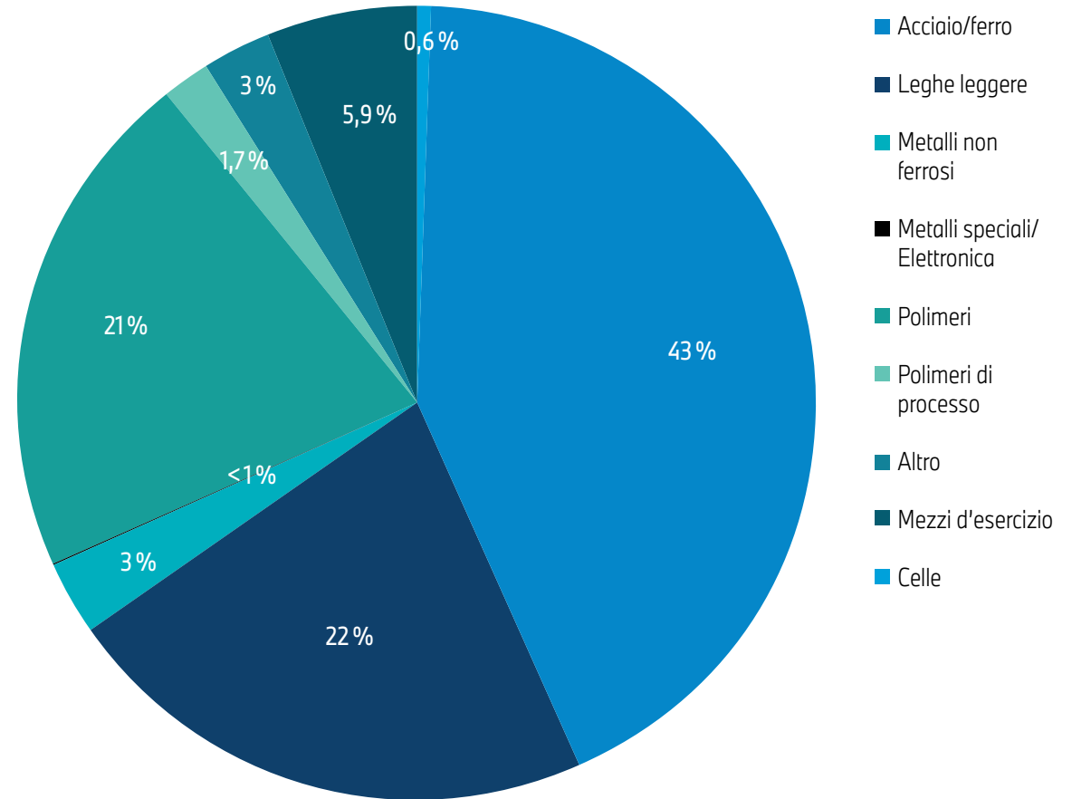
Fig. 2: Composizione dei materiali della BMW 520i berlina all'inizio della produzione. I valori indicati possono presentare differenze di arrotondamento.
