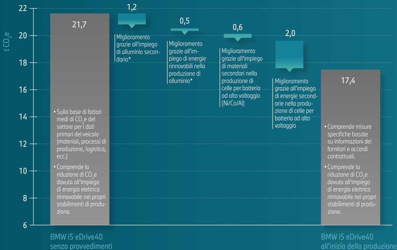
Fig. 5: Influenza degli obiettivi di sviluppo sul potenziale di riscaldamento globale della fase di produzione della BMW i5 eDrive40 Touring
